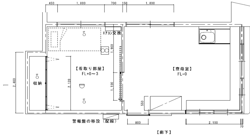
計画図
